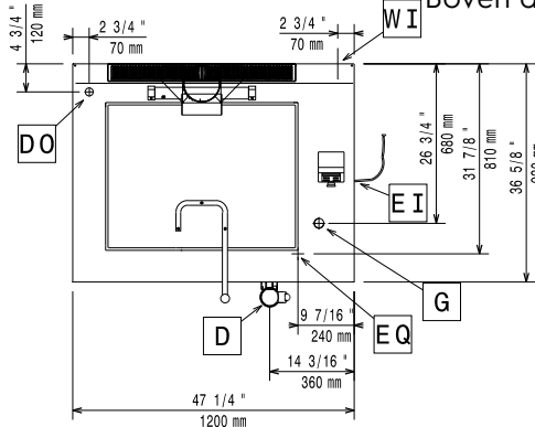
Boven aanzicht
